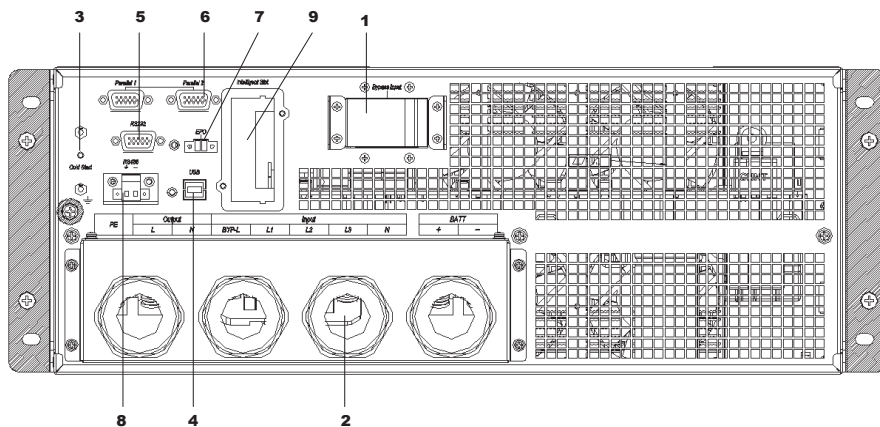
Рисунок 2.2. Вид сзади
