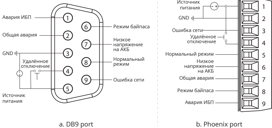
Рисунок 6.1. «Сухие» контакты
