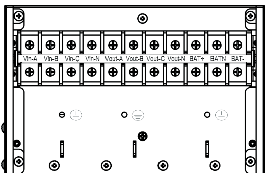
Рис. 6. 10-20 кВА
